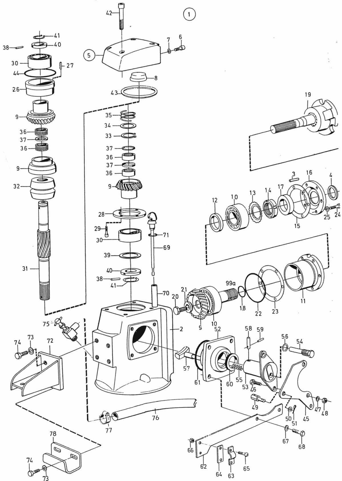
Bild 1.11, Sprängskiss 110S övre delen
