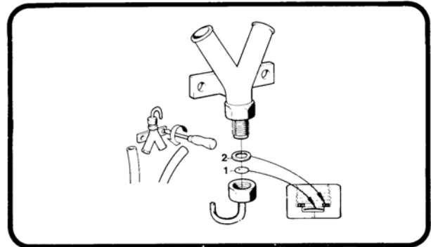
Bild 5.12, vakuumventil demontering
