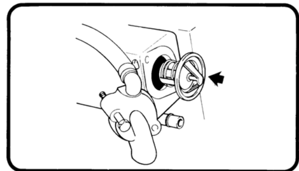
Bild 5.5, montering av termostat
