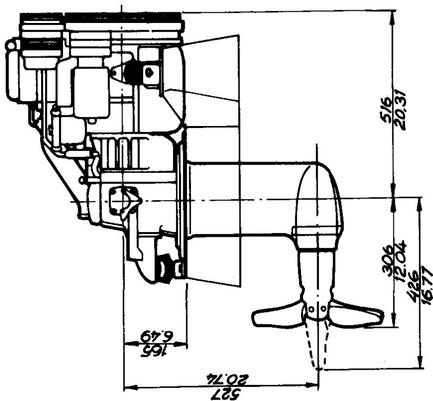
Bild 13.1, dimensioner MD5A och MD5B med110S
