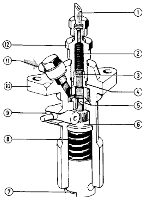
Bild 2.19 Insprutningspump på Volvo Penta MD1 (833740) är snarlik till funktion men inte identisk med den på MD5 (838150)
