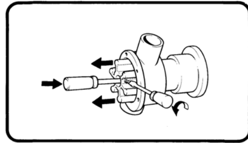
Bild 5.10, visar att man måste hålla emot så att axeln inte åker ur samtidigt som man skruvar ur medbringaraxeln.
