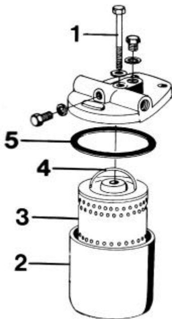
Bild 2.13, finfiltrets delar
