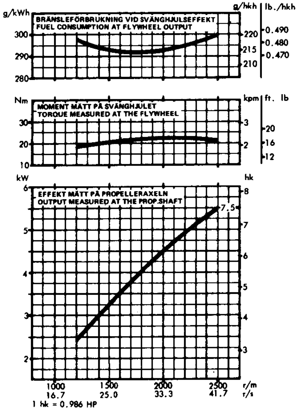
Bild 13.3, MD5A och MD5B, diagrammen visar bränsleförbrukning, vridmoment och effekt. OBS diagrammen utgår ifrån att motorn arbetar med fullgas vid alla varvtal och fås fram om man kör motorn i en bromsbänk. En marinmotor kan aldrig jobba på detta sätt så denna typ av tabell är ganska meningslös. Motorn ska, med rätt propeller, klara av att komma upp till sitt maxvarvtal på 2500 varv. Men den ska normalt köras på 70 – 80 % av maxvarvtalet, dvs 1750 – 2000 varv.
