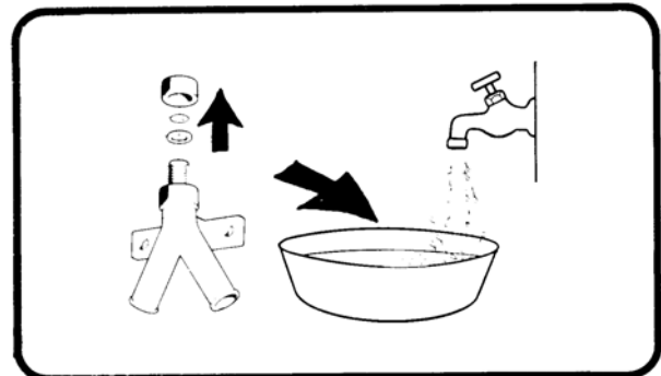
Bild 5.13, rengöring vakuumventil
