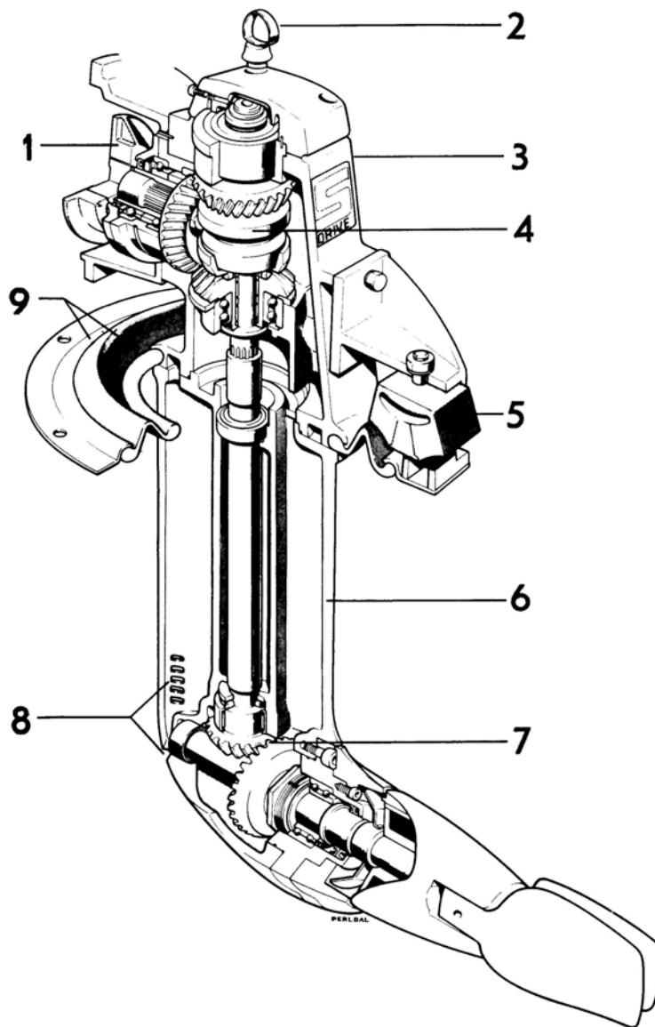
Bild 1.10, 110S Drev
