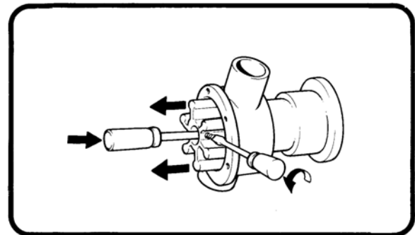
Bild 9.3, impellerbyte
